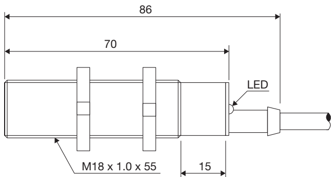
Fig. 6 Cable CA18CAF...A2IO
