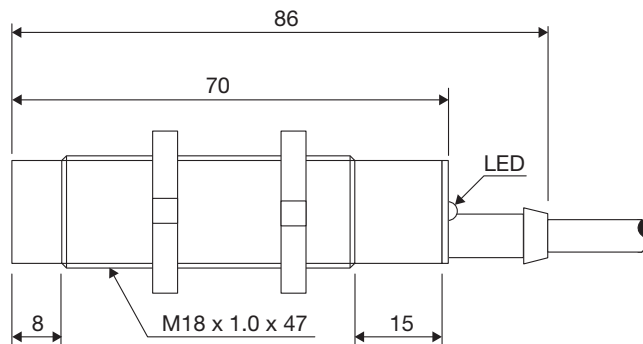
Fig. 7 Cable CA18CAN...A2IO
