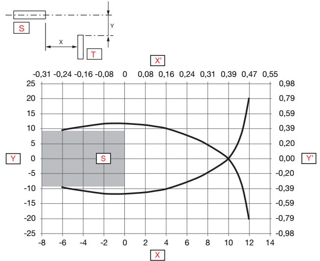
Fig. 5 No empotrado
